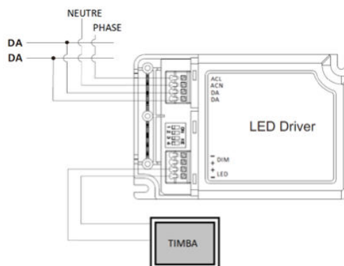
Montage pour contrôle DALI
